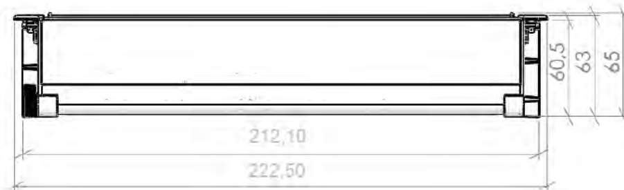
Perfil
