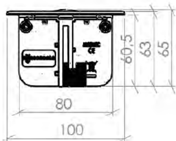
Alzado
