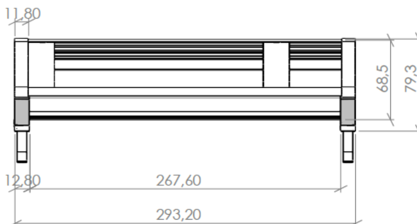
Perfil
